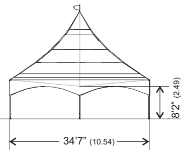
END ELEVATION
